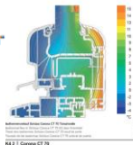
Kombischwelle nach innen öffnend Combination threshold, inward-opening Seuil combiné - ouverture vers l'intérieur Umbral combinado de apertura interior
