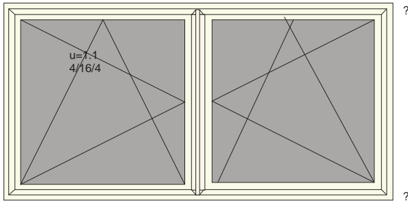
2 x draai/kiiep (Schüco handgrepen zonder slot, Winkhaus Activipilot,RCO) met hr++ glas, u=1.1, 4/16/4..
