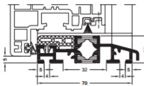
Kombischwelle nach außen öffnend Combination threshold, outward-opening Seuil combiné - ouverture vers l'extérieur Umbral combinado de apertura exterior
