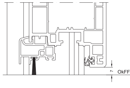
Tür ohne Schwelle Door without threshold Porte sans seuil Puerta sin umbral
