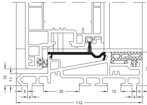
Türschwelle Accent nach außen öffnend Accent door threshold, outward-opening Seuil de porte Accent - ouverture vers l'extérieur Umbral de puerta Accent de apertura exterior
