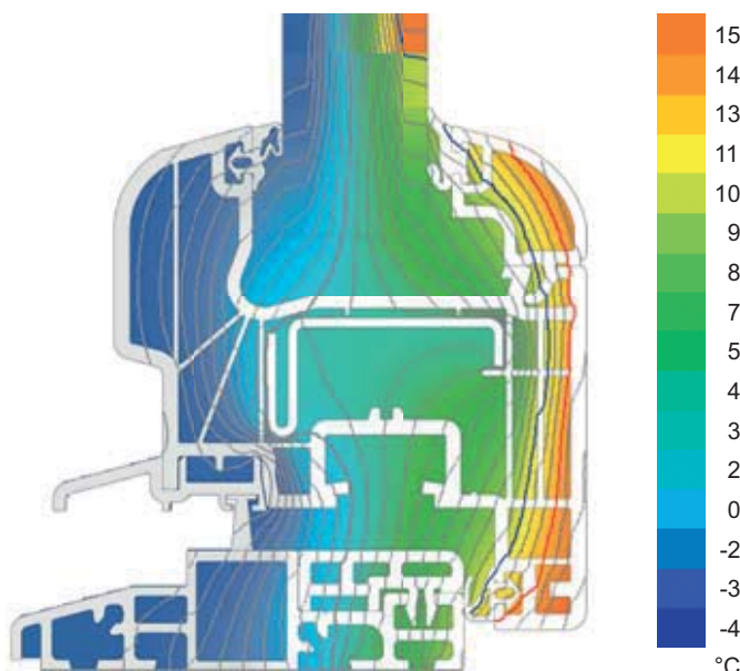
Isothermenverlauf Schüco Corona CT 70 Türschwelle Isothermal flow in Schüco Corona CT 70 AS door threshold Tracé des isothermes Schüco Corona CT 70 seuil de porte Trazado de las isotermas Schüco Corona CT 70 umbral de puerta
