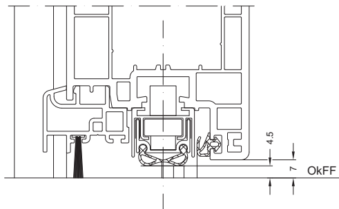
Automatische Türabdichtung nach innen öffnend Automatic door seal, inward-opening Etanchéité de porte automatique ouvrant vers l'intérieur Sellado de puerto automático de apertura interior
